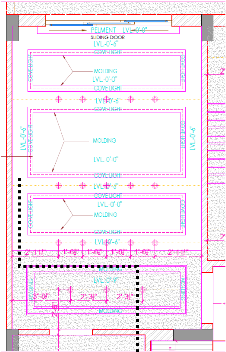
OPTION -02 -FOR BED-WALL
